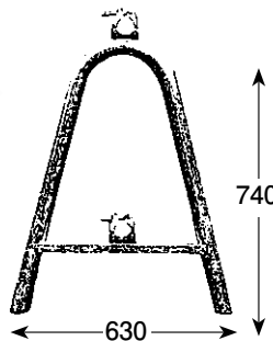
■パイプバリケード(5kg)
