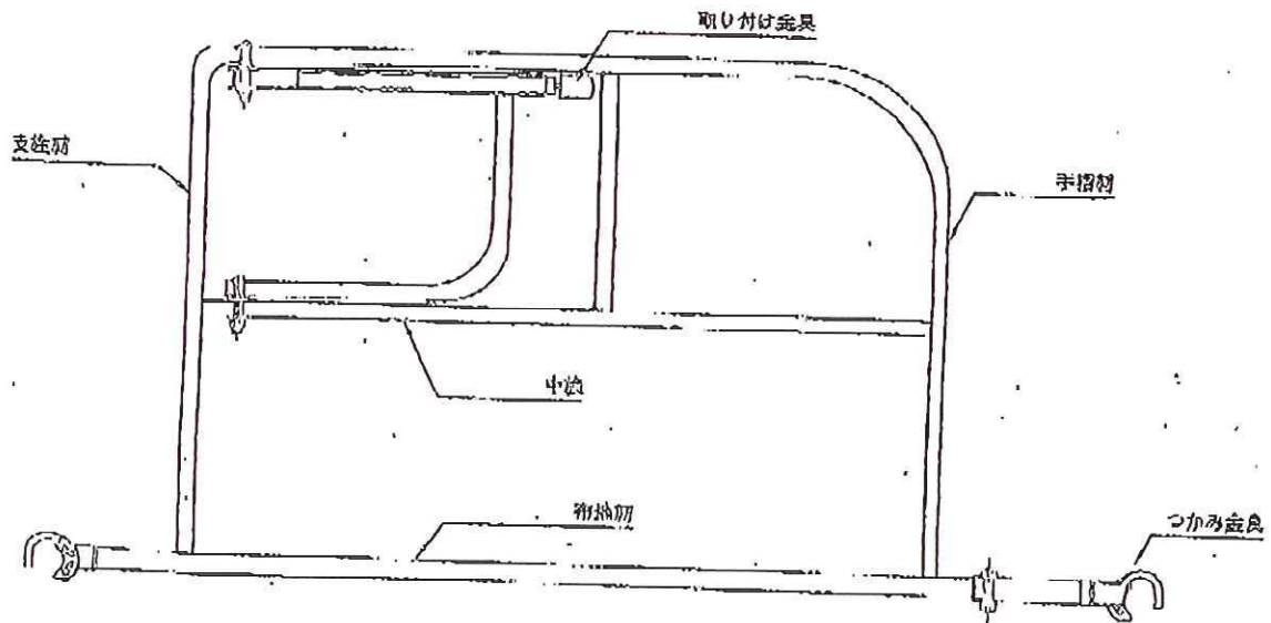
構造図
