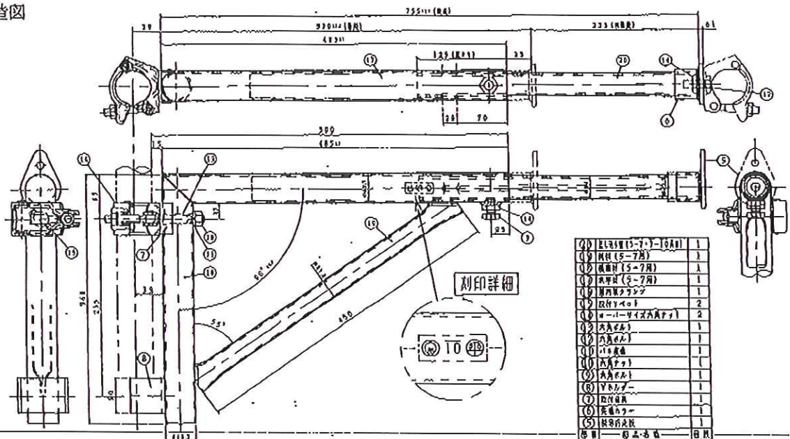
構造図
